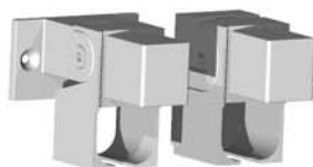
Ref. 0834 CONJUNTO BISAGRA PARA LA GUÍA DE PÉRGOLA
