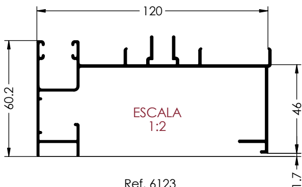
Ref. 6123 CERCOS LATERAL IZQ. CAJON MONOBLOCK
