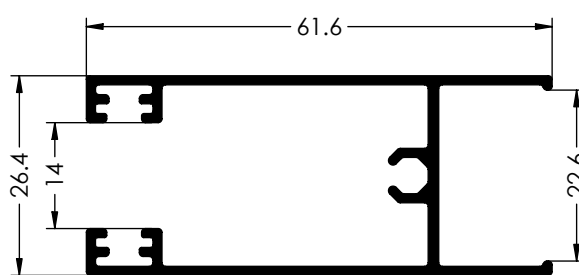
Ref. 6103B HOJA DE RUEDAS CLIMALIT
