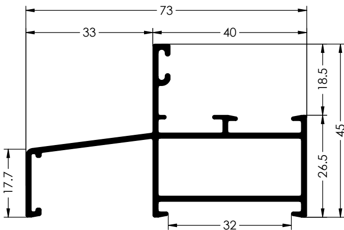
Ref. 6098 CERCO FIJO
