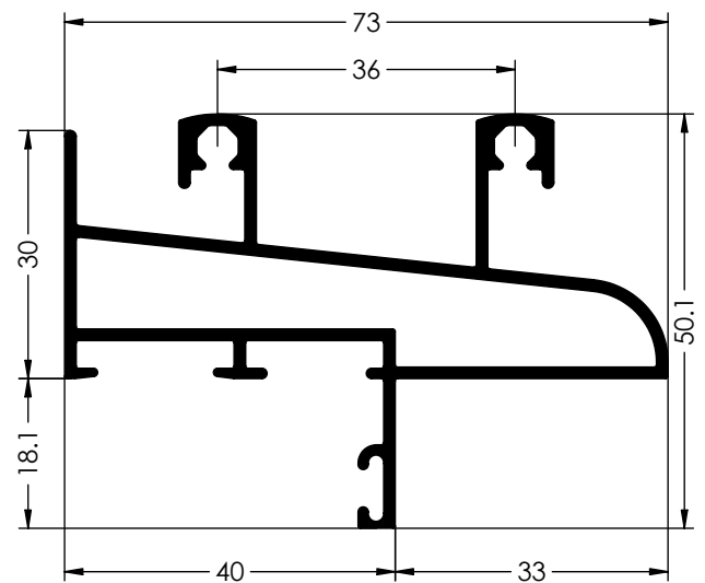
Ref. 6097 CERCO INFERIOR FIJO
