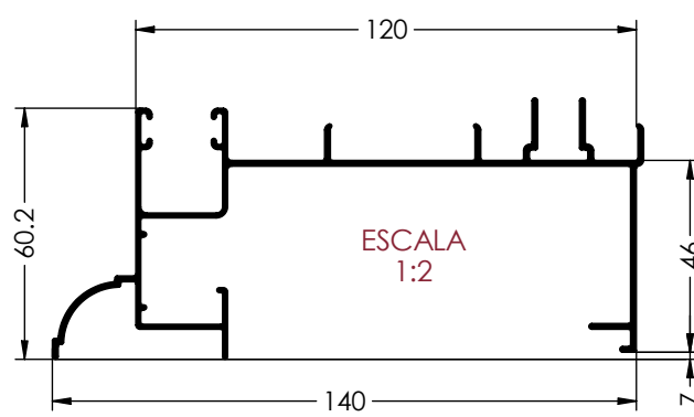
Ref. 6113 CERCOS LATERAL DCHO. CAJON MONOBLOCK
