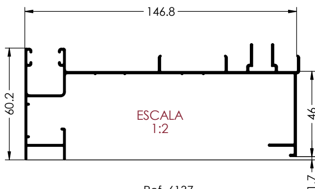
Ref. 6137 CERCOS LATERAL DCHO. CAJON MONOBLOCK
