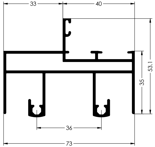
Ref. 6099 CERCO SUPERIOR FIJO INC.
