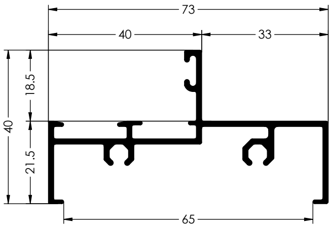
Ref. 6096 CERCO FIJO
