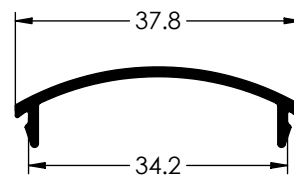
Ref. 6107 EMBELLECEDOR CERCOS LATERAL
