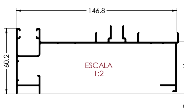
Ref. 6138 CERCOS LATERAL IZQ. CAJON MONOBLOCK
