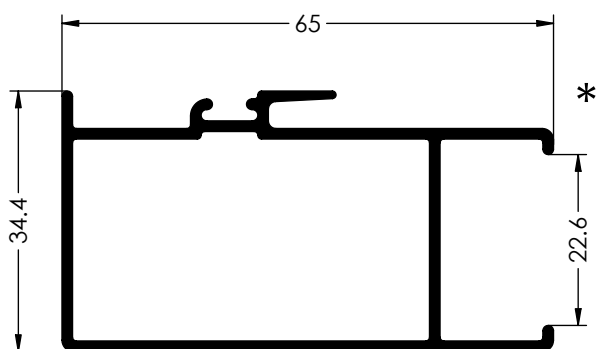
Ref. 6042 HOJA LATERAL CIERRE DE PUNTOS
