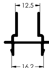
Ref. 4515 PERFIL 4 HOJAS
