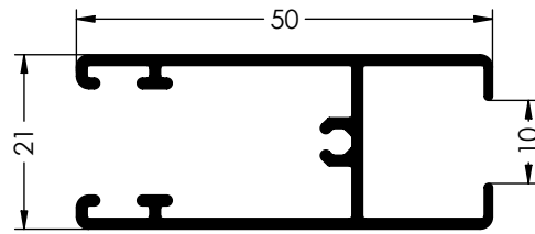
Ref. 6090 HOJA DE RUEDAS GUSANILLO MONOLITICO
