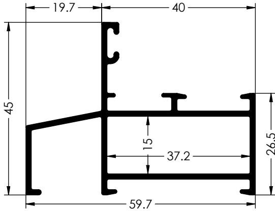
Ref. 6012 CERCOS FIJOS
