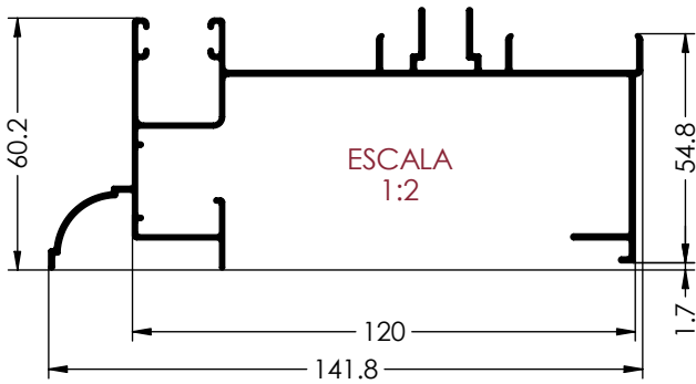
Ref. 6081 CERCOS LATERAL IZQUIERDO (MONOBLOCK)
