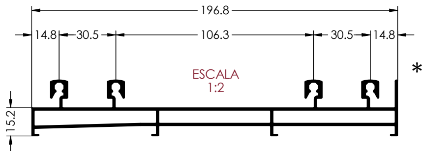
Ref. 6143 CERCO INFERIOR DOBLE
