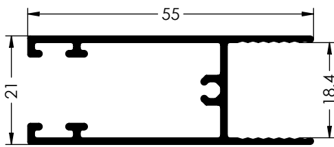
Ref. 6046 HOJA DE RUEDAS GUSANILLO
