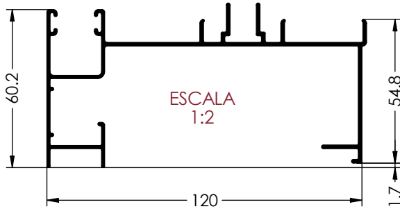
Ref. 6129 CERCOS LATERAL IZQUIERDO (MONOBLOCK)
