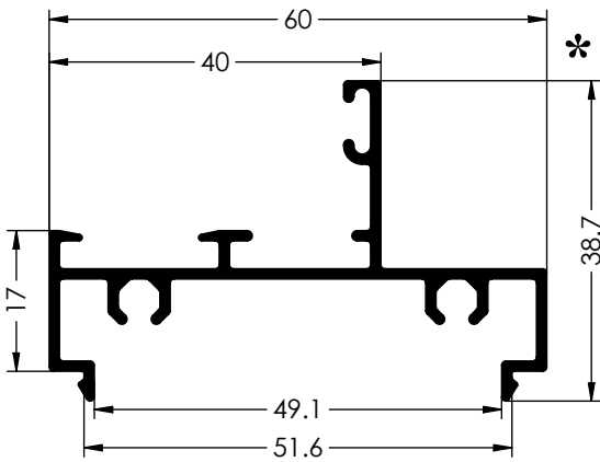
Ref. 6087 CERCOS FIJOS
