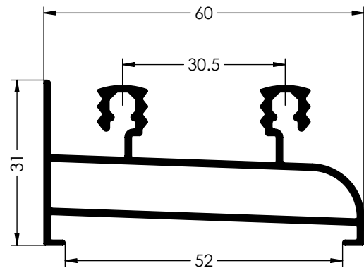
Ref. 6052 CERCOS INFERIORES TUBULARES
