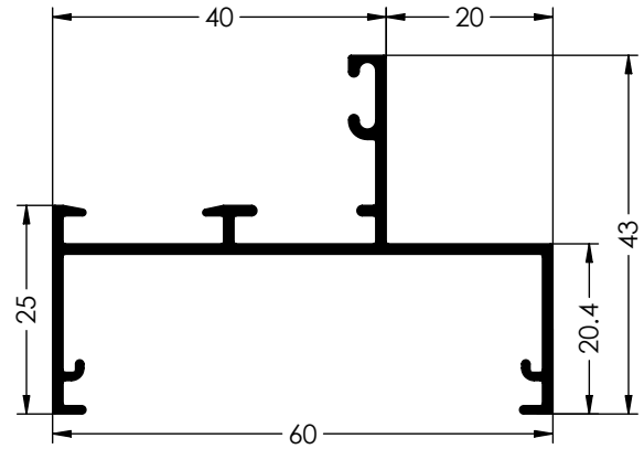
Ref. 6060 CERCOS FIJOS
